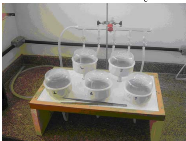
Figura 5. Aparato para a desidratação ultra-rápida desenvolvida no Laboratório de Análise de Sementes do BASEMFLORE – Embrapa Florestas.
